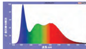
発光スペクトル (WLED)
