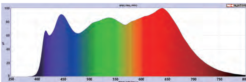
分光分布図：光子量子比率
