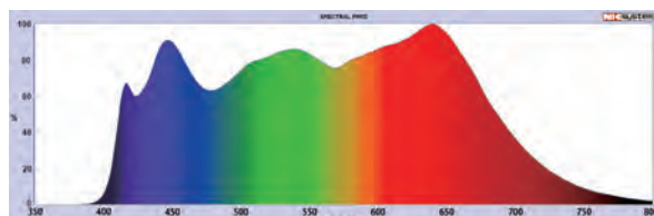
「SUNRAY LIGHT®」発光スペクトル
