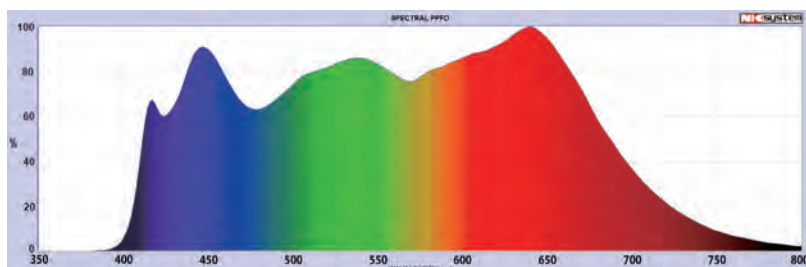
分光分布図：光子量子比率
