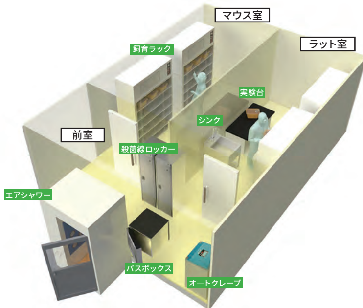
動物飼育ユニットレイアウト例
