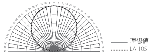
図1：コサイン応答
