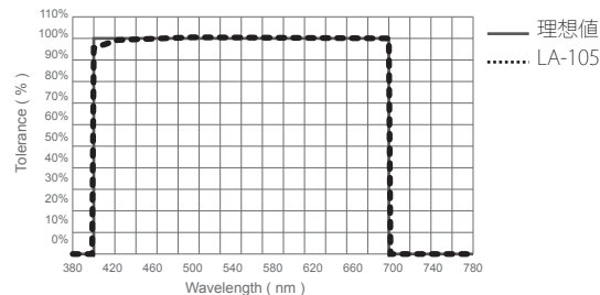
図3：光量子感度特性比較
