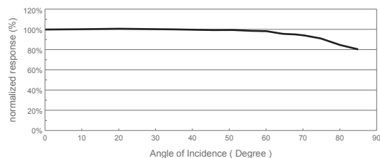
図2：コサイン補正
