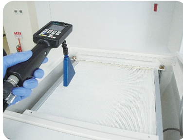
HEPAフィルタ性能試験(透過率試験)
